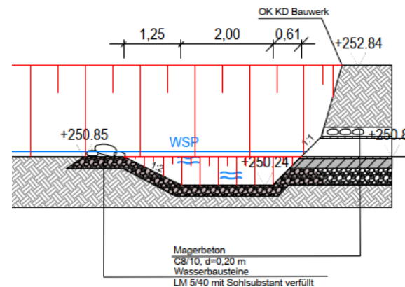
Schnitt BB Umgestaltung Zulauf Winterbergbach DN 400
