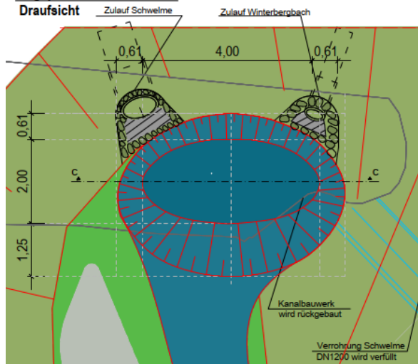
Lageplanausschnitt Draufsicht
