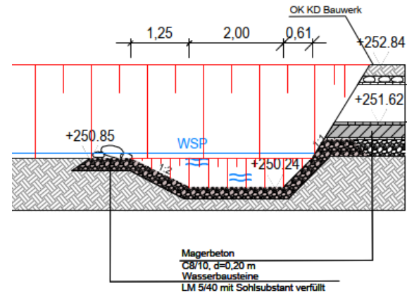
Schnitt BB Umgestaltung Zulauf Winterbergbach DN 400
