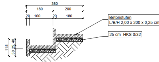
Detail A-A M 1:50
