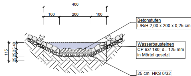
Detail A-A M 1:50
