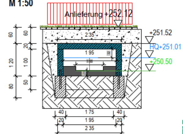
Darstellung Auslauf M 1:50
