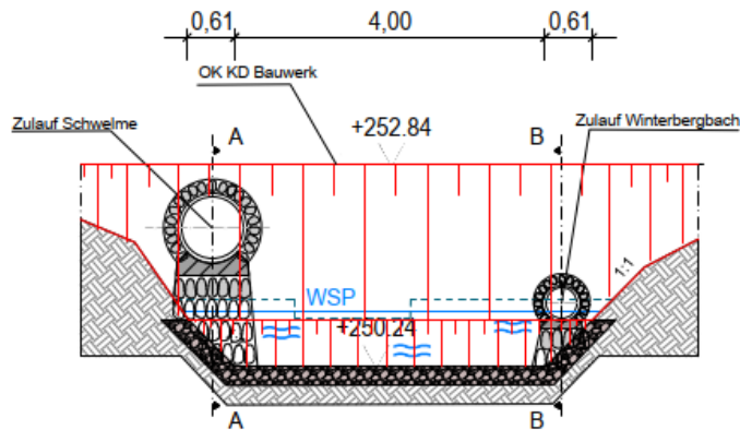
Schnitt CC Vorderansicht
