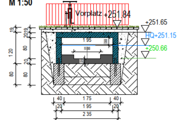
Darstellung Einlauf M 1:50
