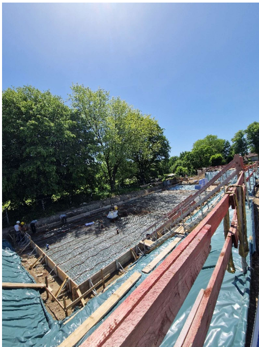
Verlegung untere Bewehrungslage
