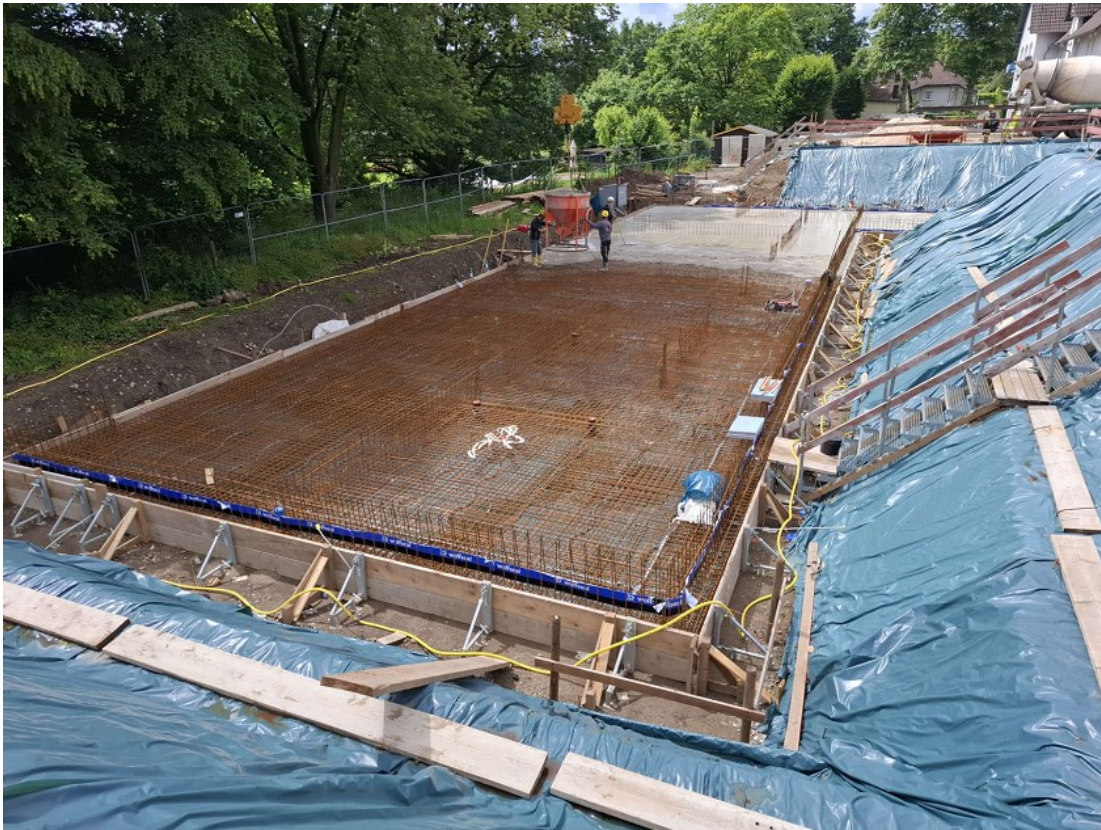
Betonieren der Bodenplatte Untergeschoss
