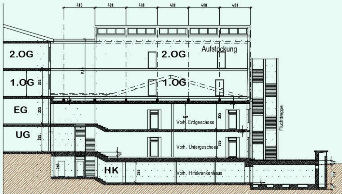
LÄNGSSCHNITT
