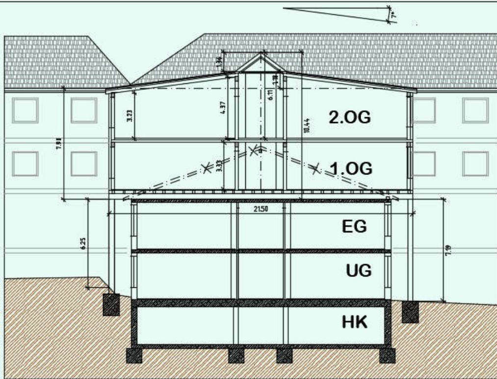
QUERSCHNITT
